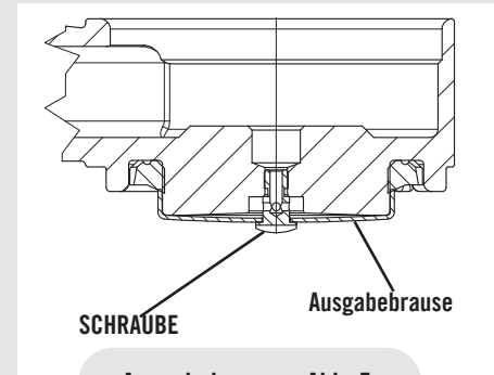
Ausgabebräuse - Abb. 5
