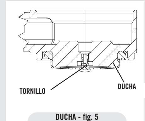
DUCHA - fig. 5
