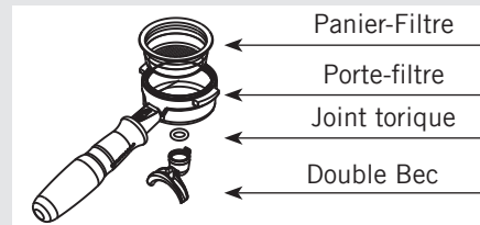
Illustration 6 - Porte-filtre - Voir part. 4, Ill. 1 ou 3
