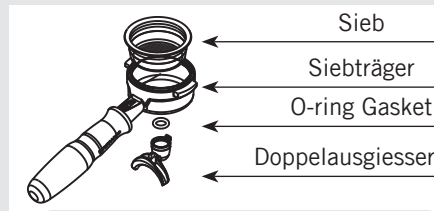
Abb. 6 - Filterrahmen (siehe 4 Abb. 1 oder 3)
